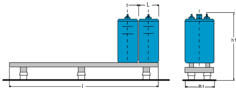
Podstawa jednorzędowa
