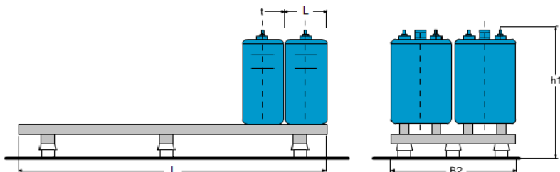
Podstawa dwurzędowa
